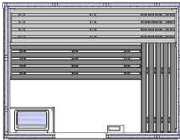
D2535 3-5 bathers 2170 x 1660 x 1950mm
